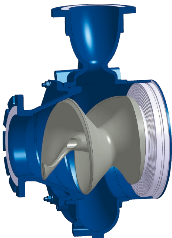
Section d'une pompe à vis centrifuge de Hidrostat
